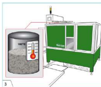
3 - Нагревание измельченной смеси для стерилизации при помощи микроволнового излучения
